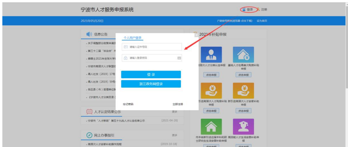
1-2 用户登录图
